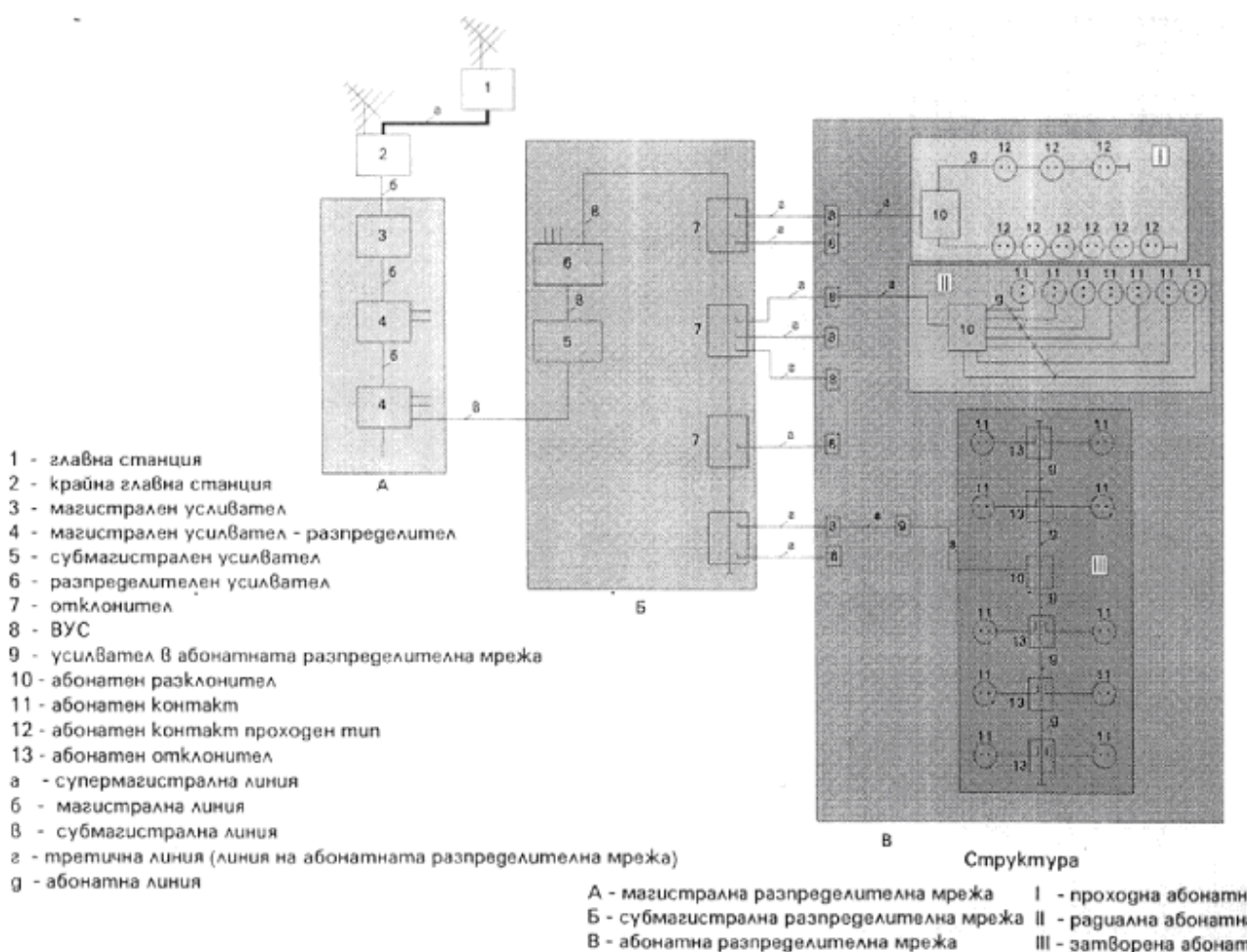
Фиг. 1. Примерна обобщена схема на кабелна мрежа
